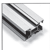
■ ZÁKLADNÍ SVISLÝ PROFIL
