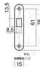
protiplech
