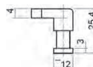
zamykácí háček
