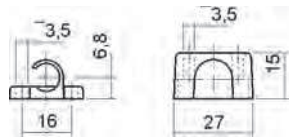
držák koncový
