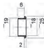
rozeta Ø 18 mm
